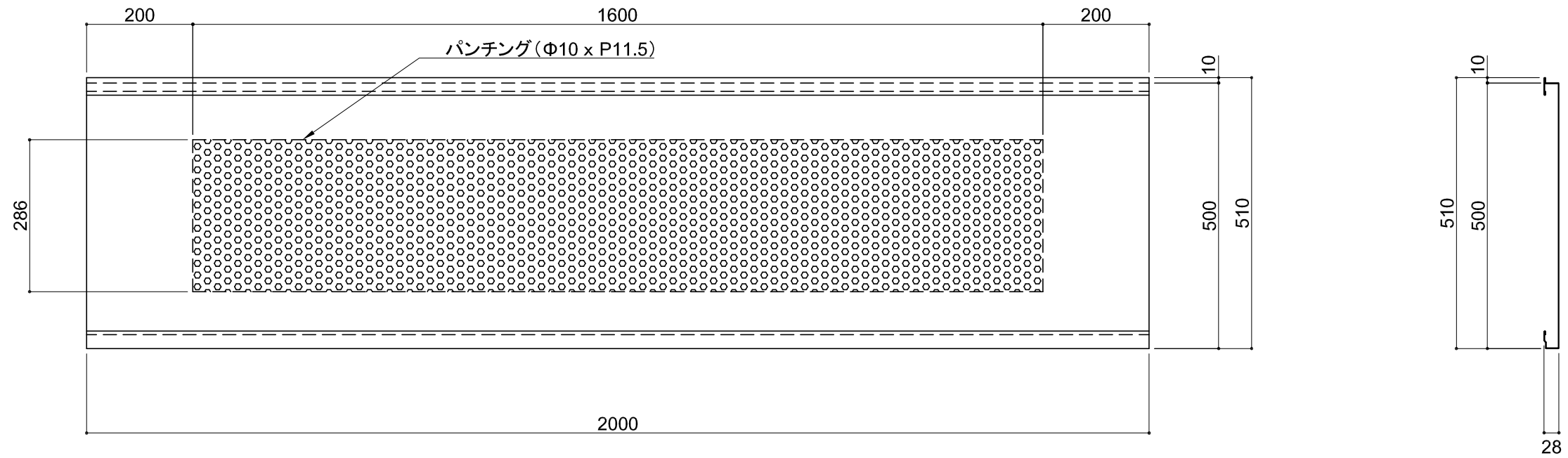
背面図(S=1/10)
