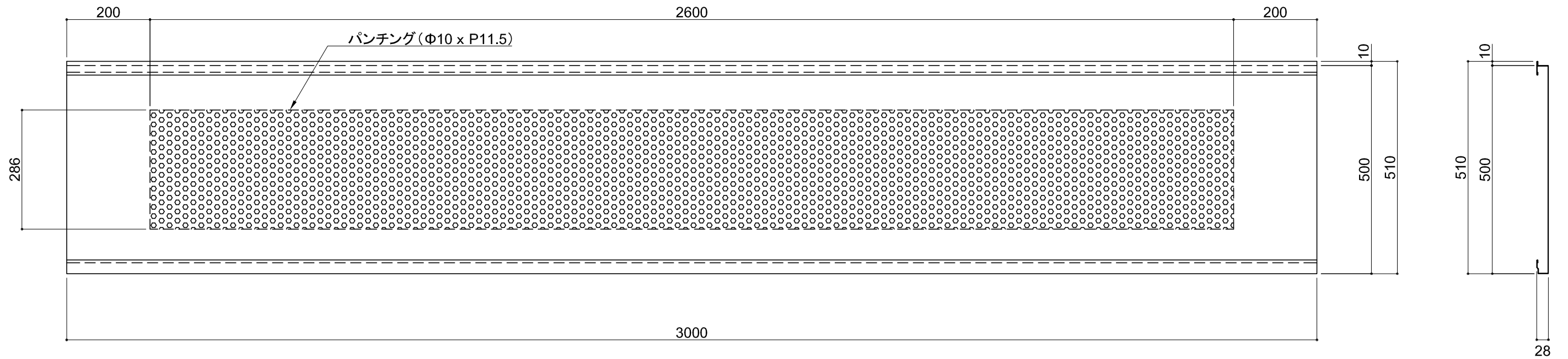
背面図(S=1/10)
