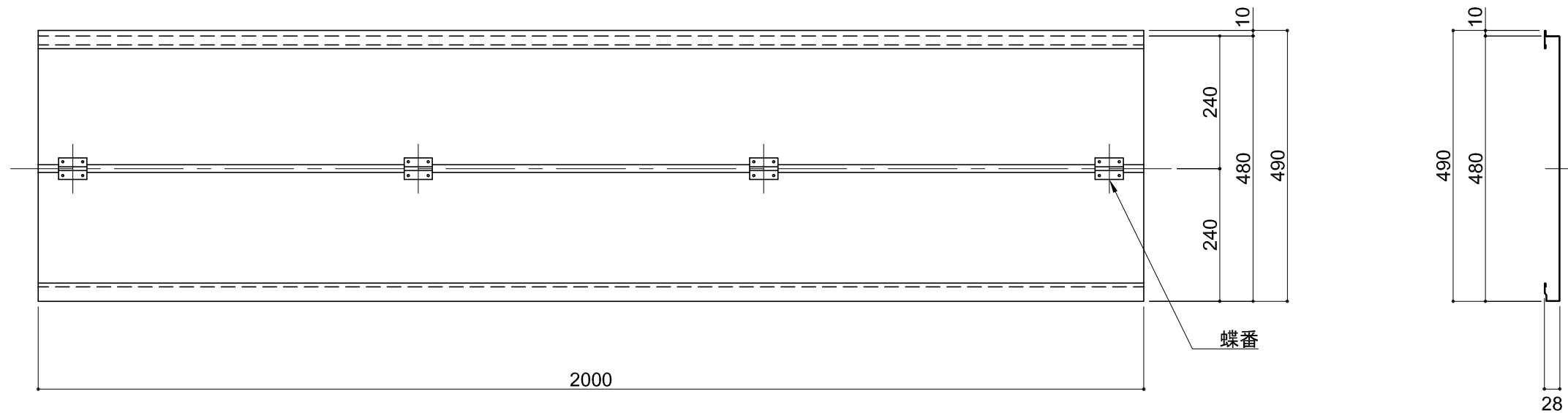
断面詳細図(S=1/2)
