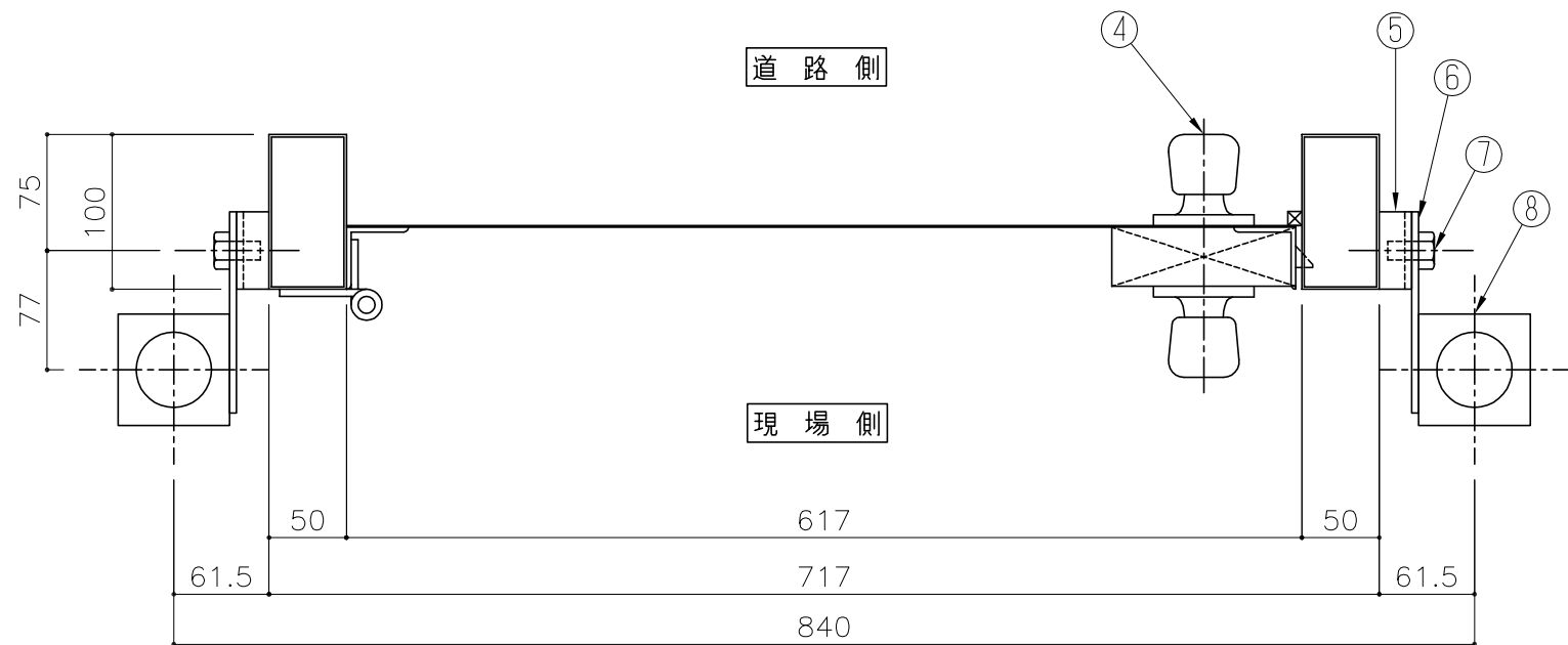
A-A断面図 (S=1/5)
