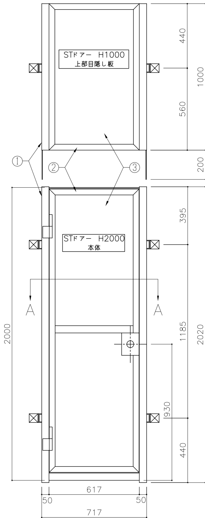
背面図
