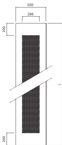
■ 正面図
