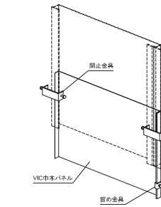
■ 設置イメージ図
