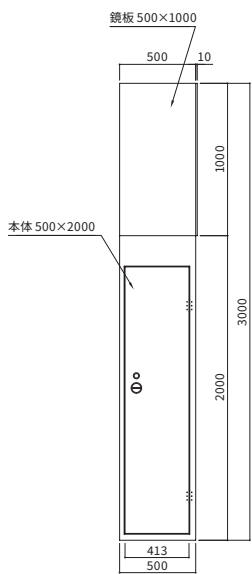
■ 正面図
