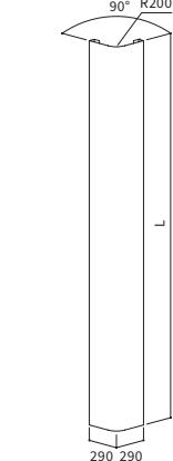
■ 正面図
