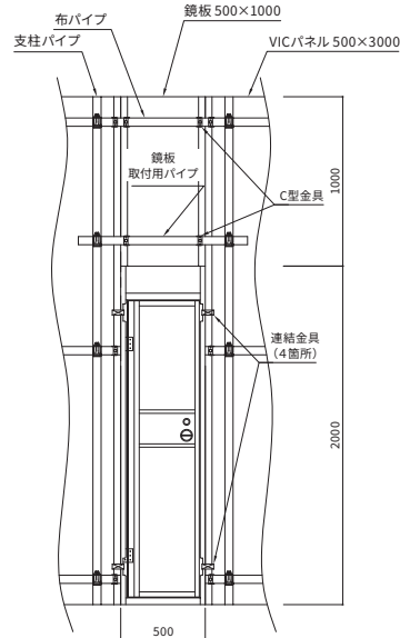
■ 裏面図
