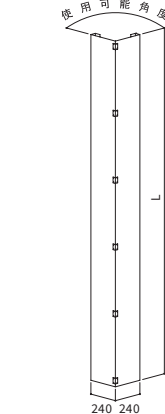
■ 正面図
