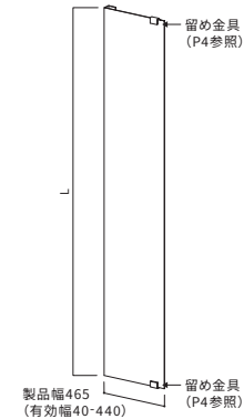
■ 正面図
