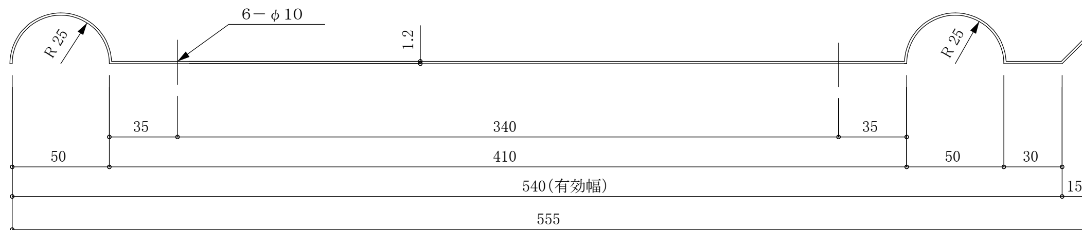
断面詳細図 (S=1/2)
