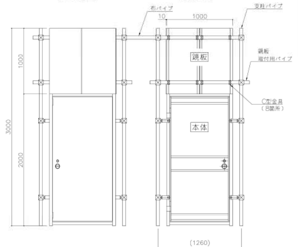
■正面図
