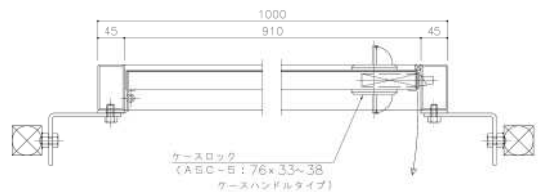
■正面図
