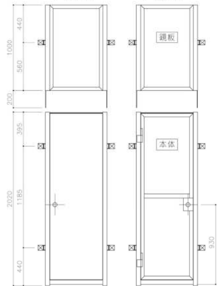
■正面図
